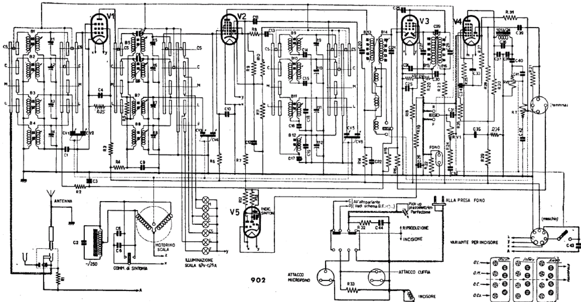
PHONOLA RADIO - Mod. 902 - Lunghie da 2000 a 927 m, medie da 600 a 187 m, corte da 51,7 a 23 m, cortissime da 23,4 a 11,4 m. Media frequenza 470 kc/s. Posizione compensatori v. schema mod. 625. Potenza d'uscita 10 W. Consumo 120 W. (Per valvole v. schema BF, per tensioni v. tabella mod. 625).
